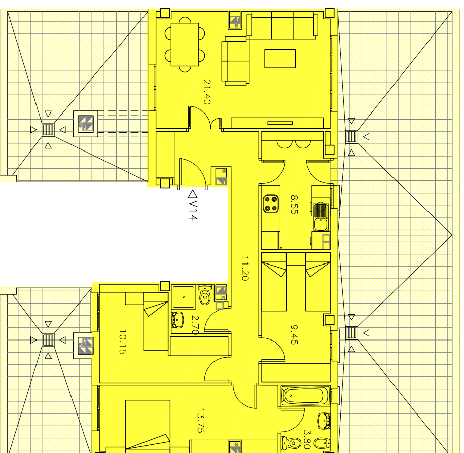
V14. SUP. ÚTIL TOTAL=81.00m2 TERRAZAS EN USUFRUCTO 54,35_24,85_14,65 (total=93,85)
